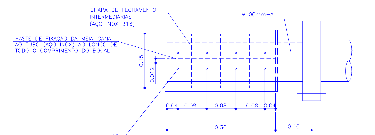
OBS: TODAS AS PEÇAS DOS BOCAIS DIFUSORES CONFECCIONADAS EM AÇO 316
