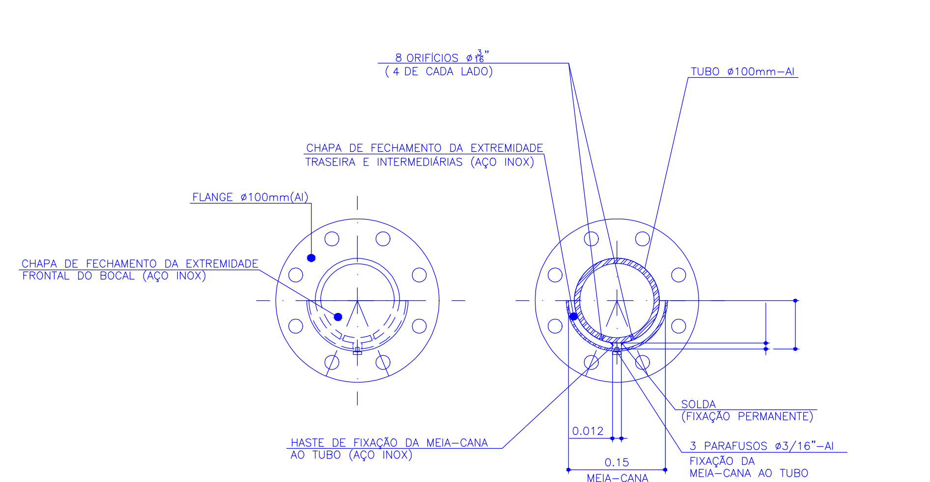
CORTE D-D
