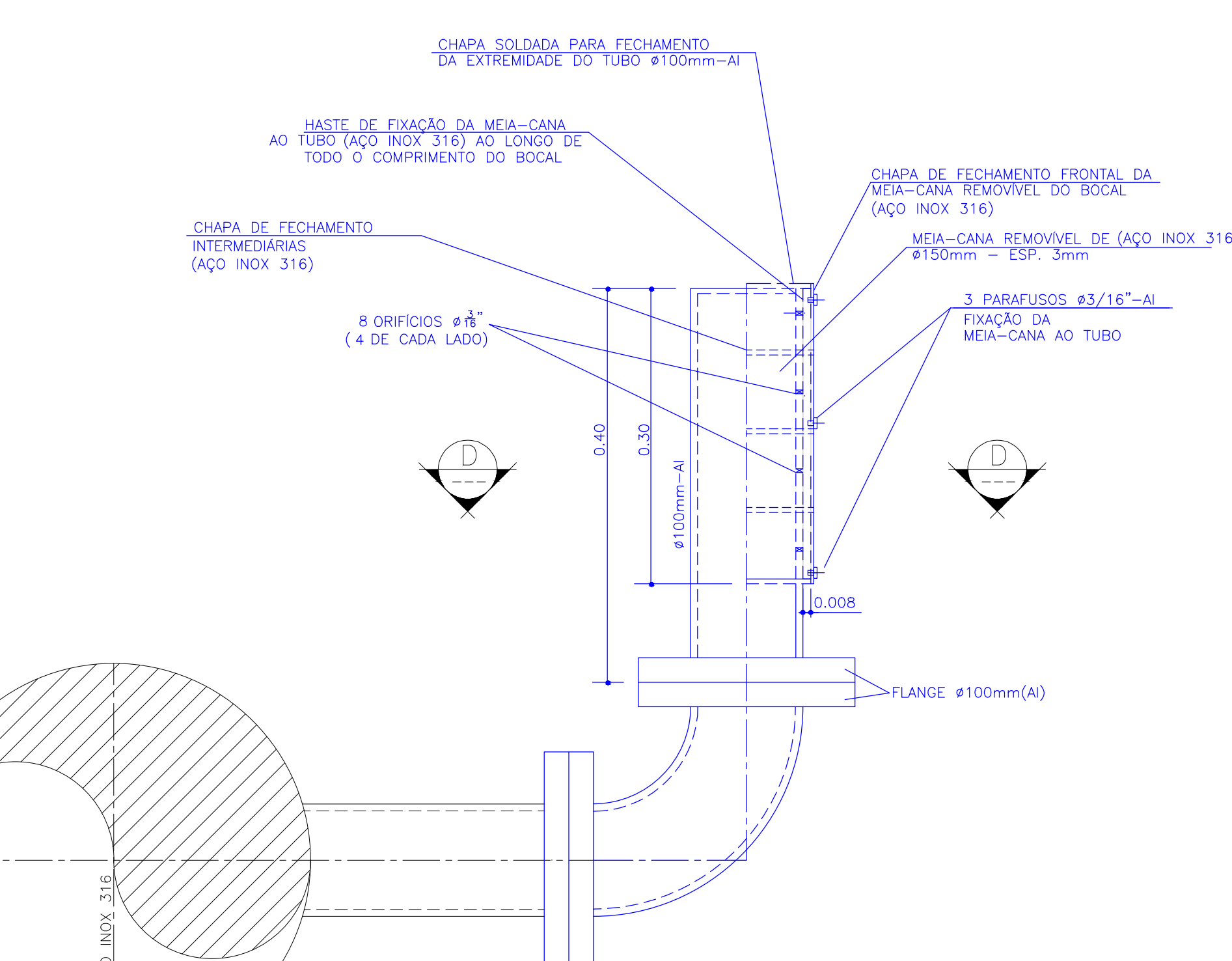
OBS: TODAS AS PEÇAS DOS BOCAIS DIFUSORES CONFECCIONADAS EM AÇO 316
