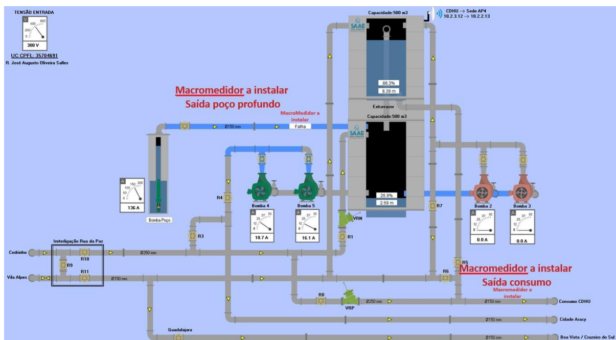
Tela de monitoramento do centro de reservação CDHU - Sistema Scada SAAE São Carlos
