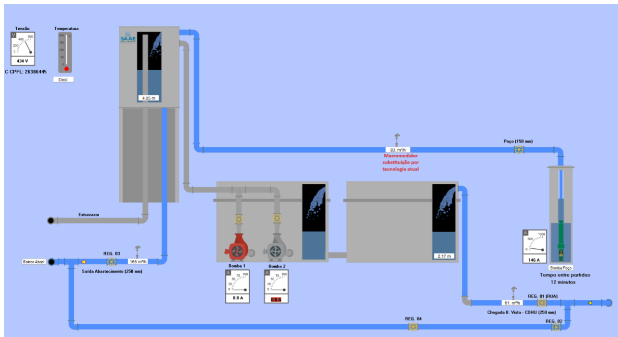
Tela de monitoramento do Poço Cruzeiro do Sul - Sistema Scada SAAE São Carlos
