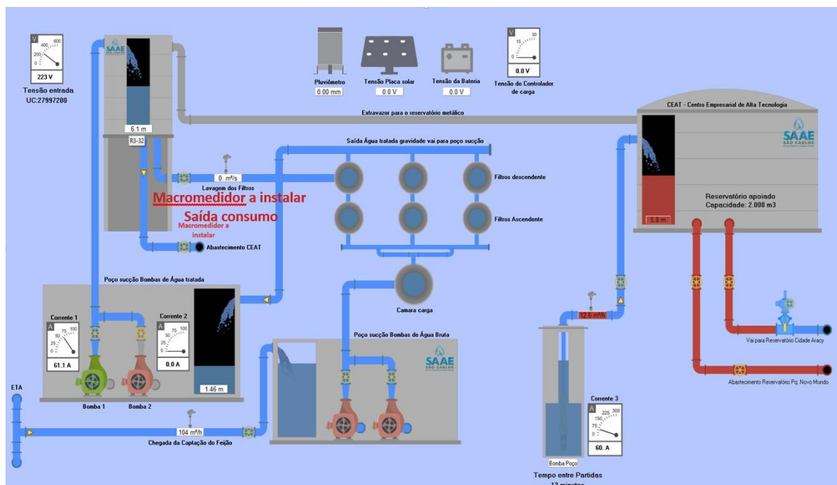
Tela de monitoramento do centro de reservação CEAT - Sistema Scada SAAE São Carlos
