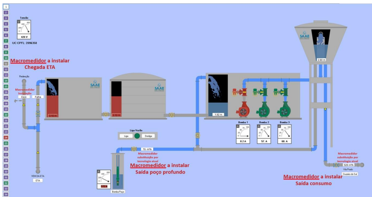
Tela de monitoramento do centro de reservação Boa Vista - Sistema Scada SAAE São Carlos
