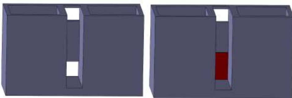
Figura 01: à esquerda, estrutura em alvenaria apresentando a entrada e descarga. À direita, com a comporta antiga (em vermelho) montada na alvenaria
