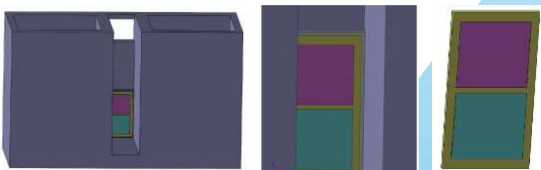
Figura 03: fixação da nova comporta (representação à direita) à moldura através de parafusos de aço inox
